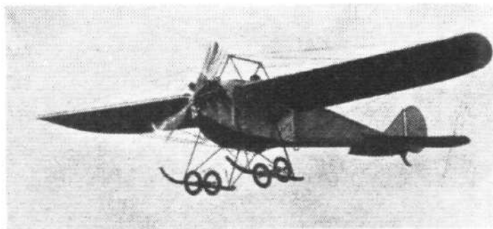
No 5 Monoplane (R.E.P.) 1912 No 7 Monoplane (Gnome) 1912
